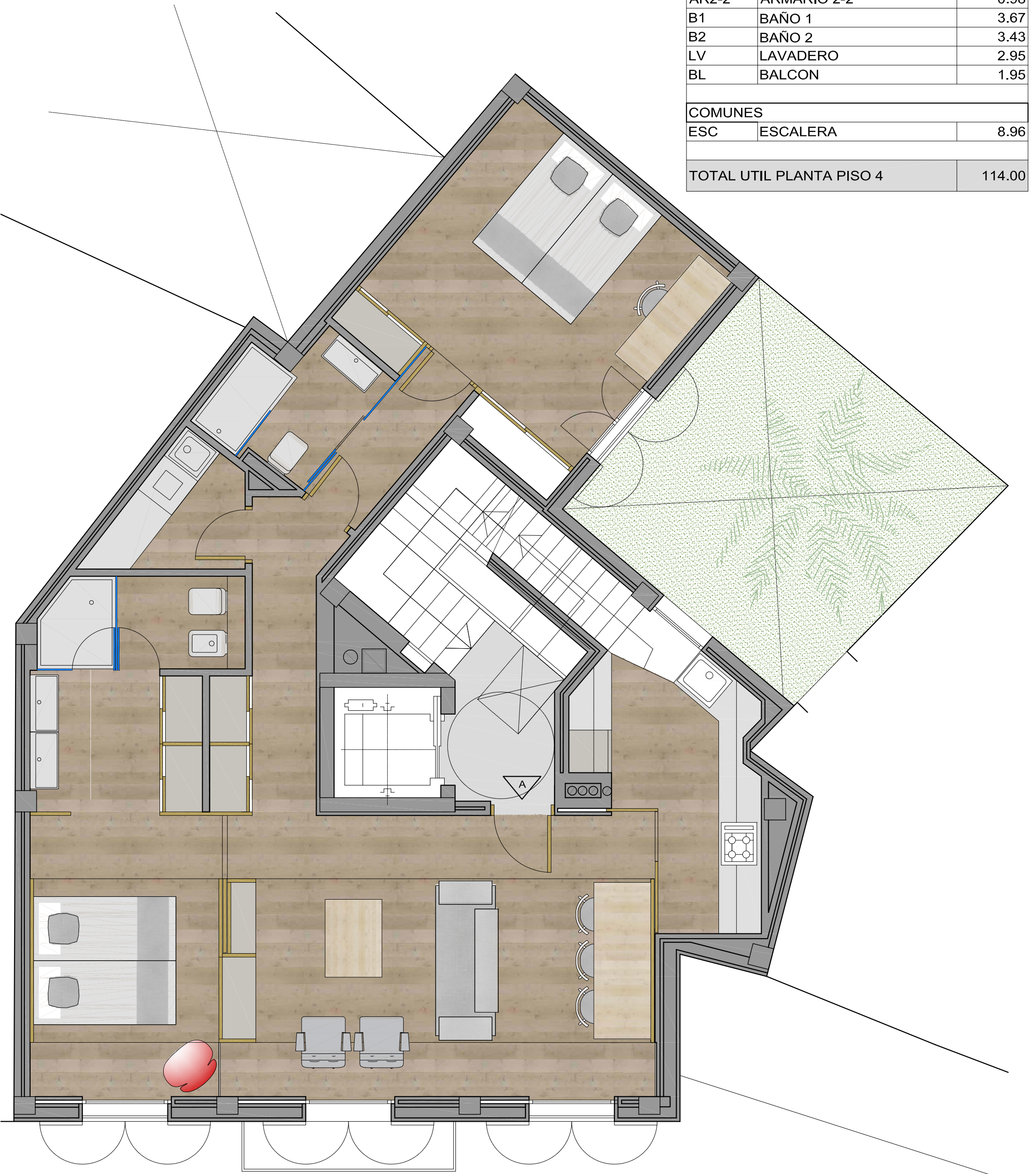
PLANTA PISO 4º PLAÇA PORTA STA. CATALINA
