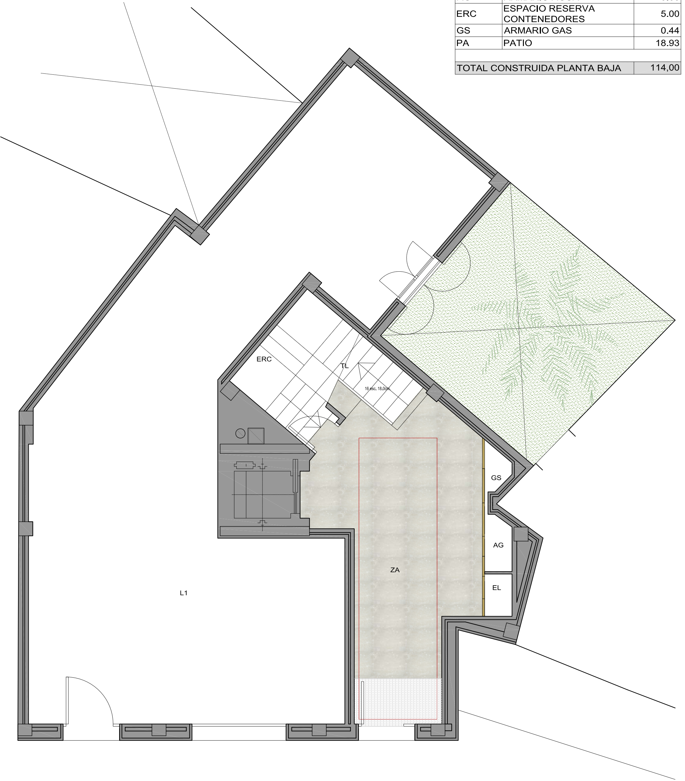
PLANTA BAJA
