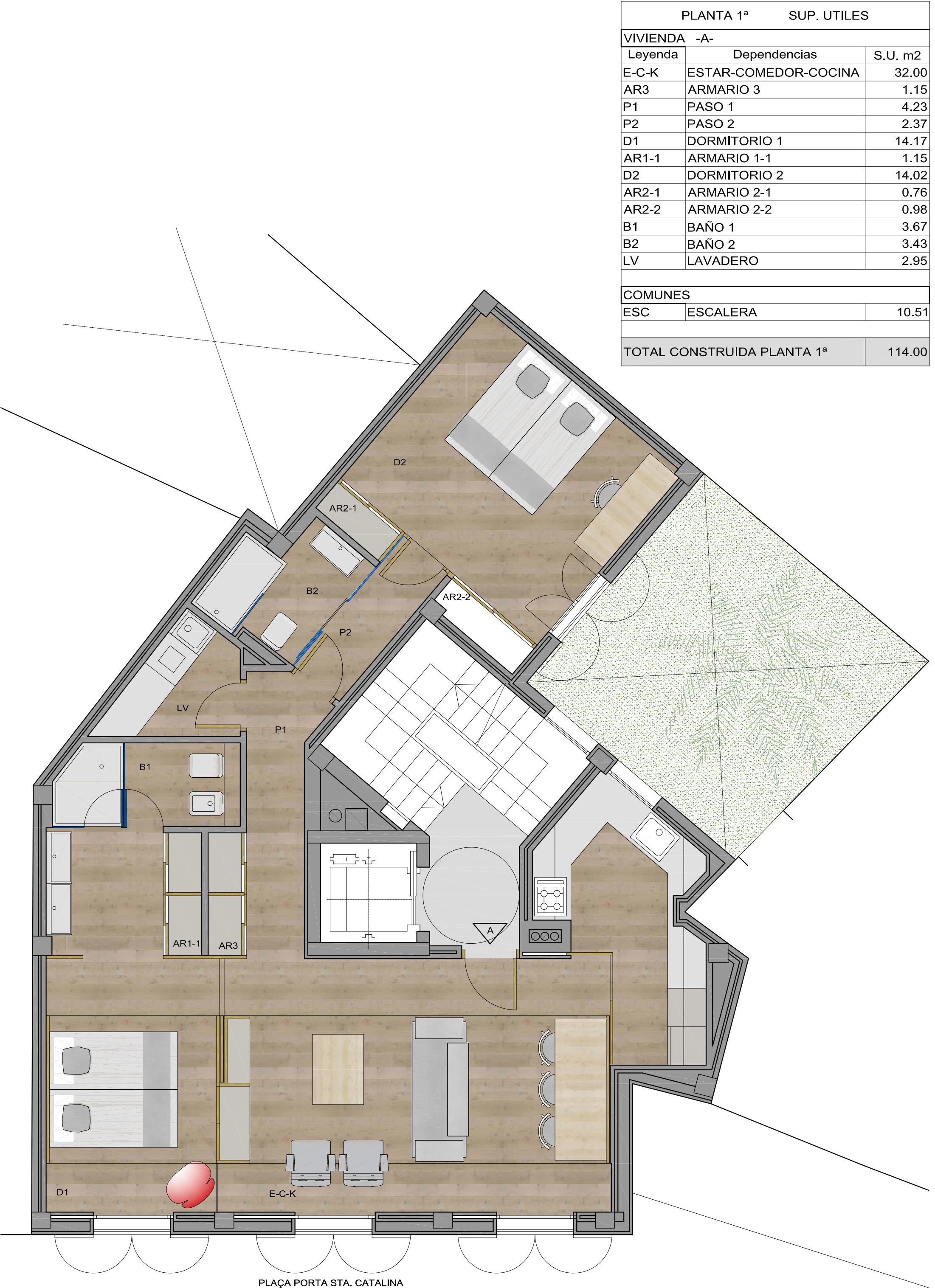
PLANTA PISO 1º PLAÇA PORTA STA. CATALINA
